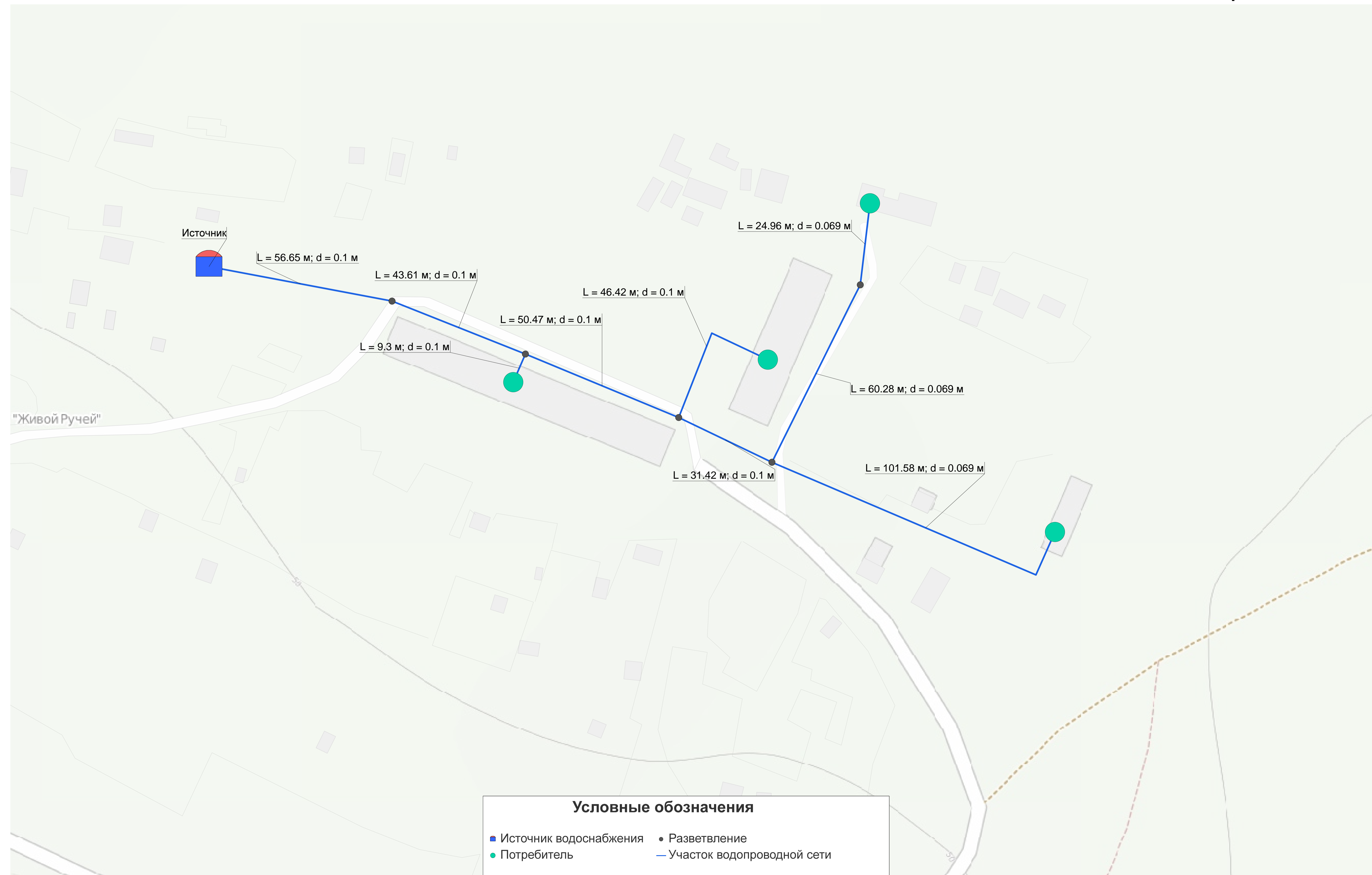
Схема водоснабжения п. дом отдыха Живой ручей
